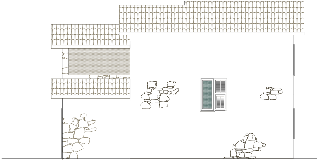
Prospetto nord
