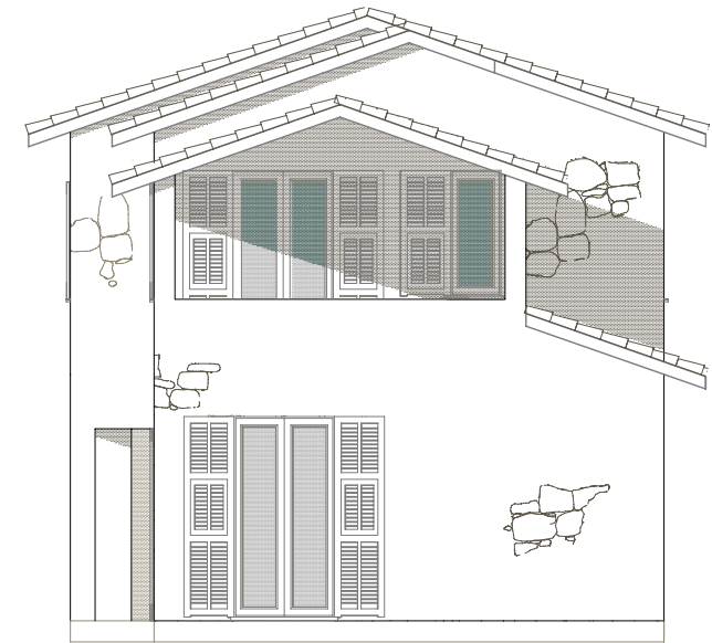
Prospetto ovest
