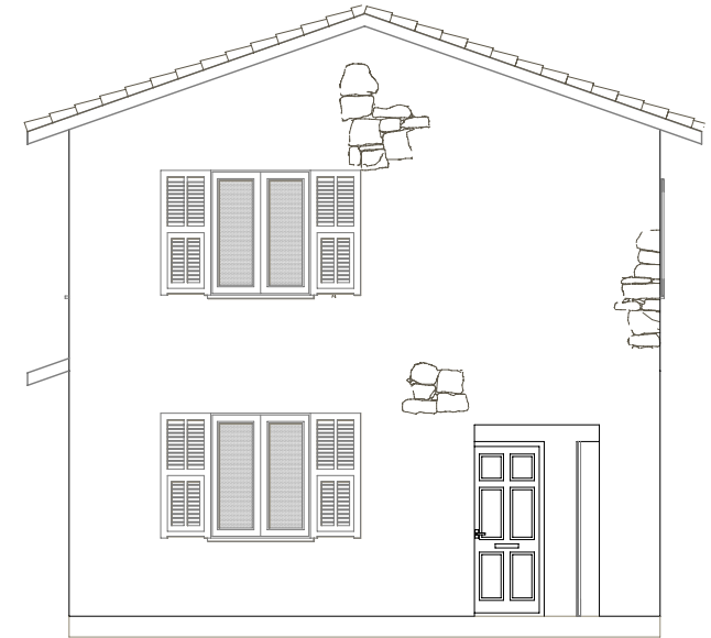
Prospetto est
