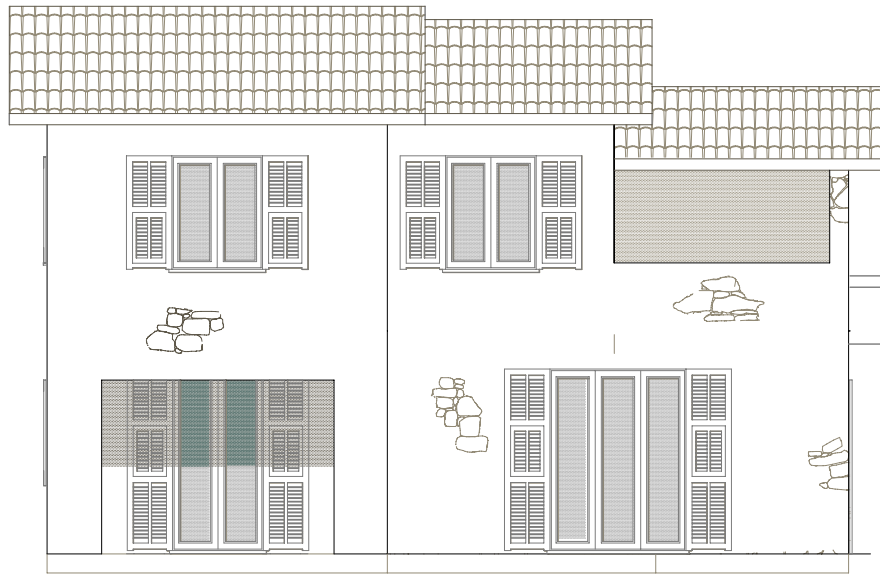
Prospetto sud
